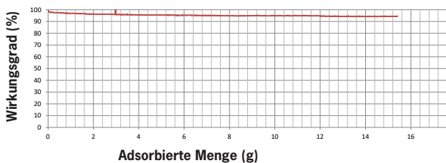
Wirkungsgrad vs. adsorbierte Menge
