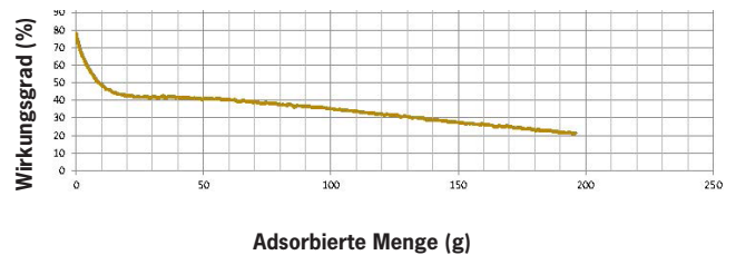
Wirkungsgrad vs. adsorbierte Menge
