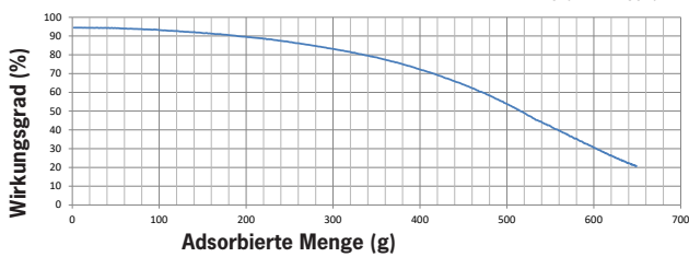
Wirkungsgrad vs. adsorbierte Menge
