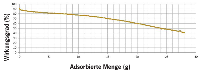
Wirkungsgrad vs. adsorbierte Menge
