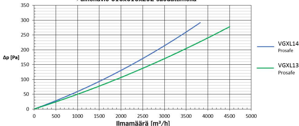
Painehäviö 610x610x292 suodattimella
