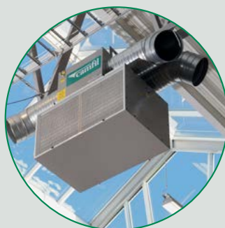
OPHÆNG TIL LOFTS-MONTERING (HORISONTAL), 4 STK. PER ENHED
